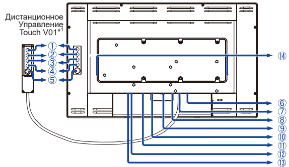
<Вид сзади>
